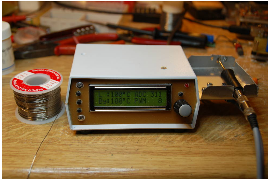
Ansicht der Lötstation
